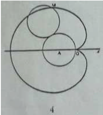
schéma 4 : cardioïde, extraite du Dictionnaire des mathématiques, Paris, PUF, 1979
