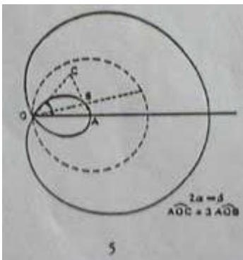
schéma 5 : Limaçon de Pascal : cas particulier de cardioïde découvert par Etienne Pascal, père de Blaise Pascal. Le nom du père est caché dedans.
